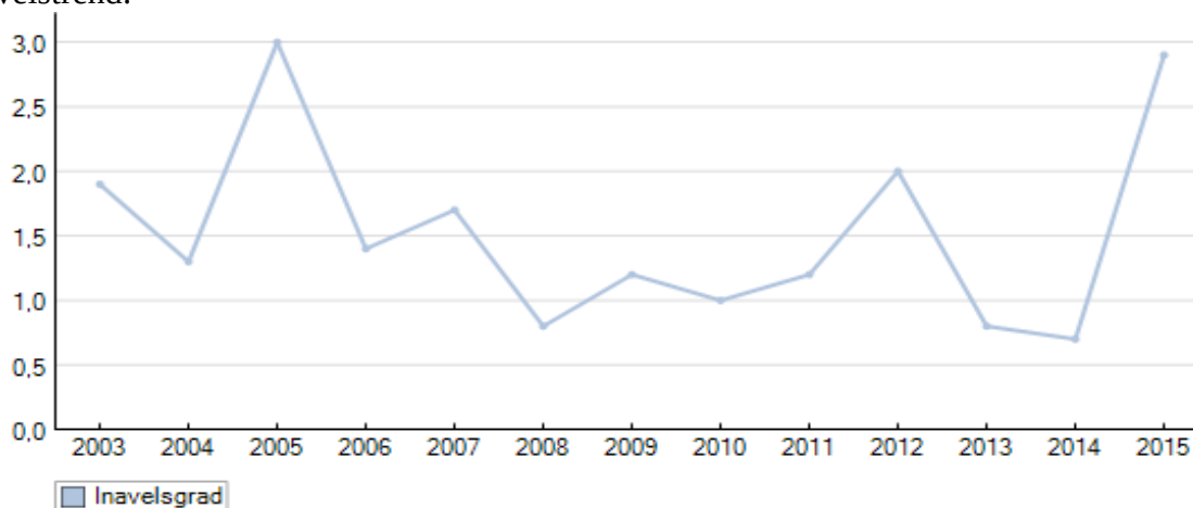
Bild 2. Inavelsgraden beräknad på 5 generationer är med god marginal under önskade 2,5 %, med undantag 2005 och 2015.
